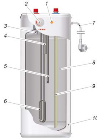
Şek 1: OW-E tipi depolu elektrikli su ısıtıcı konstrüksiyonu
